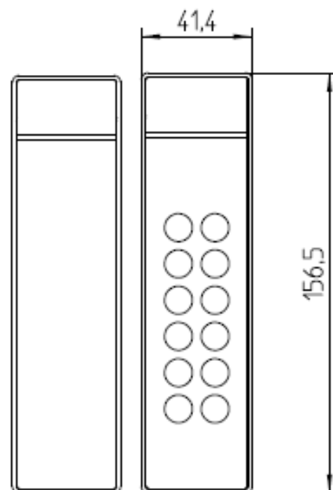
Buitenbehuizing LSW
