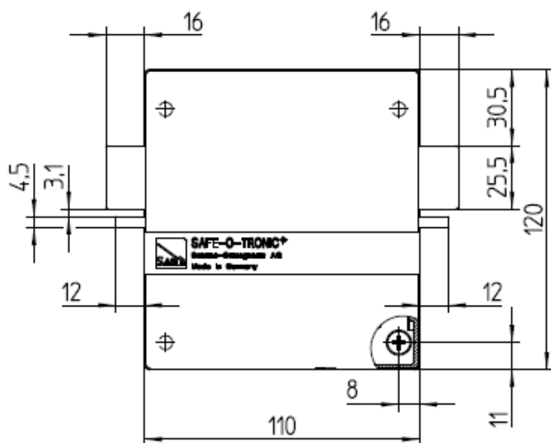
Binnenbehuizing LSW
